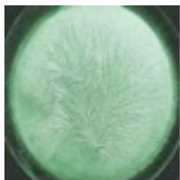
appel kristallisatie met CuCl2
